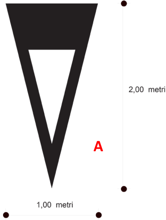
Figura Il 442/a RIDOTTO Reg. - C.d.S. - Art. 148 SIMBOLO SULLA PAVIMENTAZIONE Triangolo elongato complementare del segnale verticale DARE LA PRECEDENZA SU STRADE DI TIPO E-F
